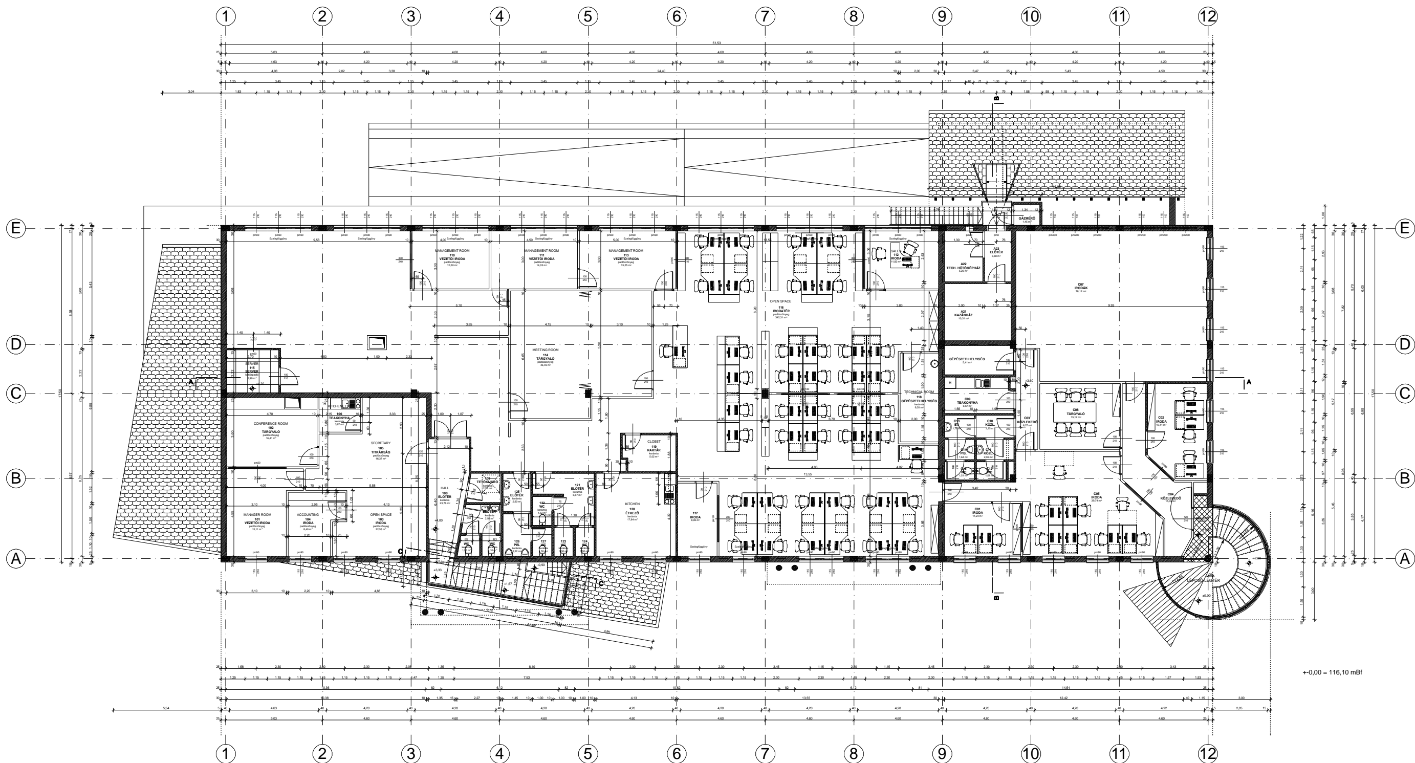
MAGNUM IRODAHÁZ EMELETI ALAPRAJZ - TERVEZETT ALAPRAJZ - M=1:100
